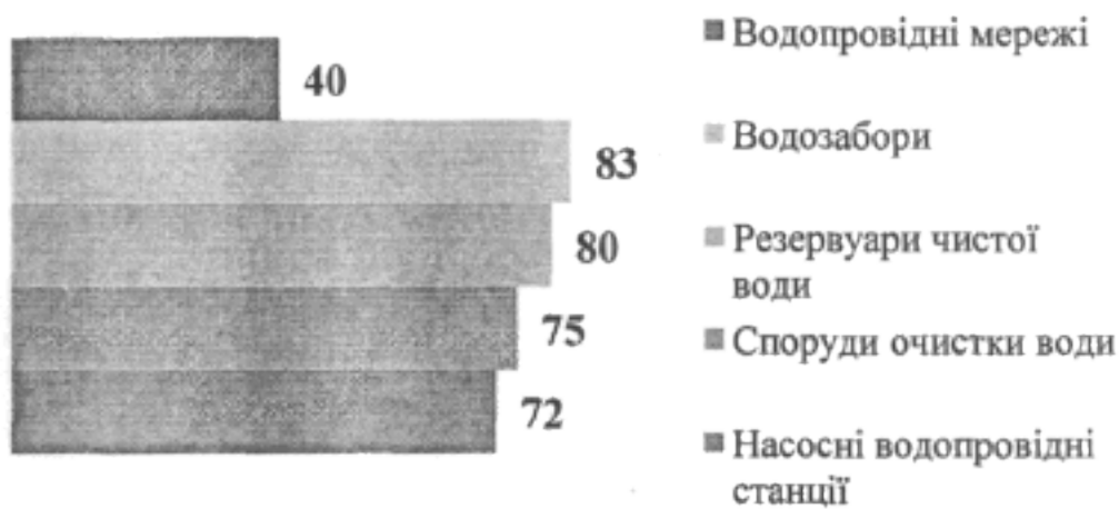
Рівень зношеності основних об'єктів та споруд водопровідного господарства, %
