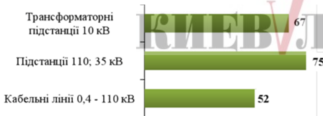
Рівень зношеності електричних мереж станом на 01.10.2017, %
